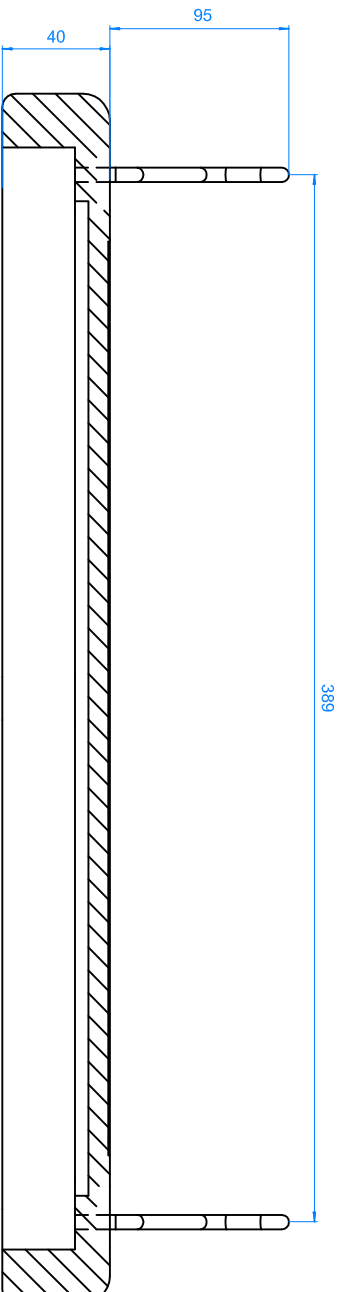
SEZIONE A-A 1:2
